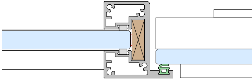
CONNEXION DE GLASS SLIM AVEC UN VERRE DE 10 OU 12MM (3/8" OU 1/2") AU CADRE DE PORTE GLASS SLIM
