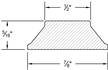
#1 7/8" OG MUNTIN
